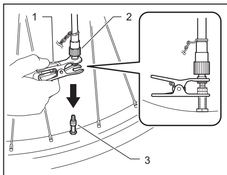
► 1. Adaptador de válvula inglesa 2. Mandril neumático 3. Vástago de la válvula
