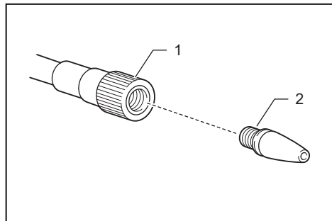
► 1. Mandril neumático 2. Adaptador cónico
